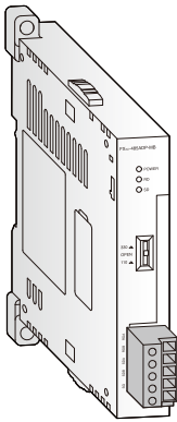
FX3U-485ADP-MB
